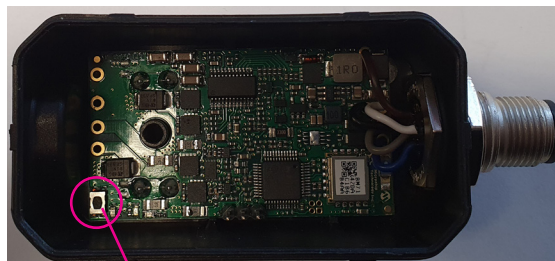
Konfigurationstaste
