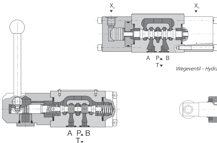
Wegeventil - Manuell betätigt (RPR3-06)
