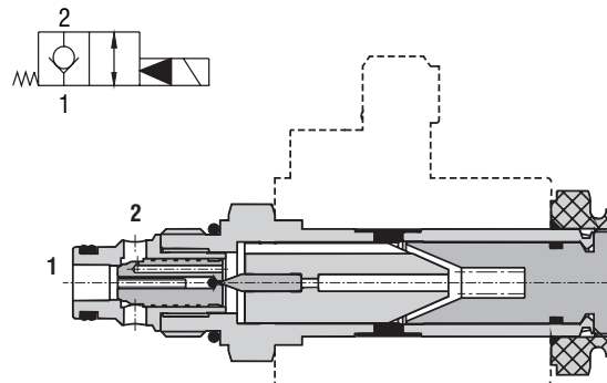
Eingebautes Kegelsitzventil, vorgesteuert
