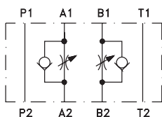
Drosselrückschlagventil 2VS3-06
