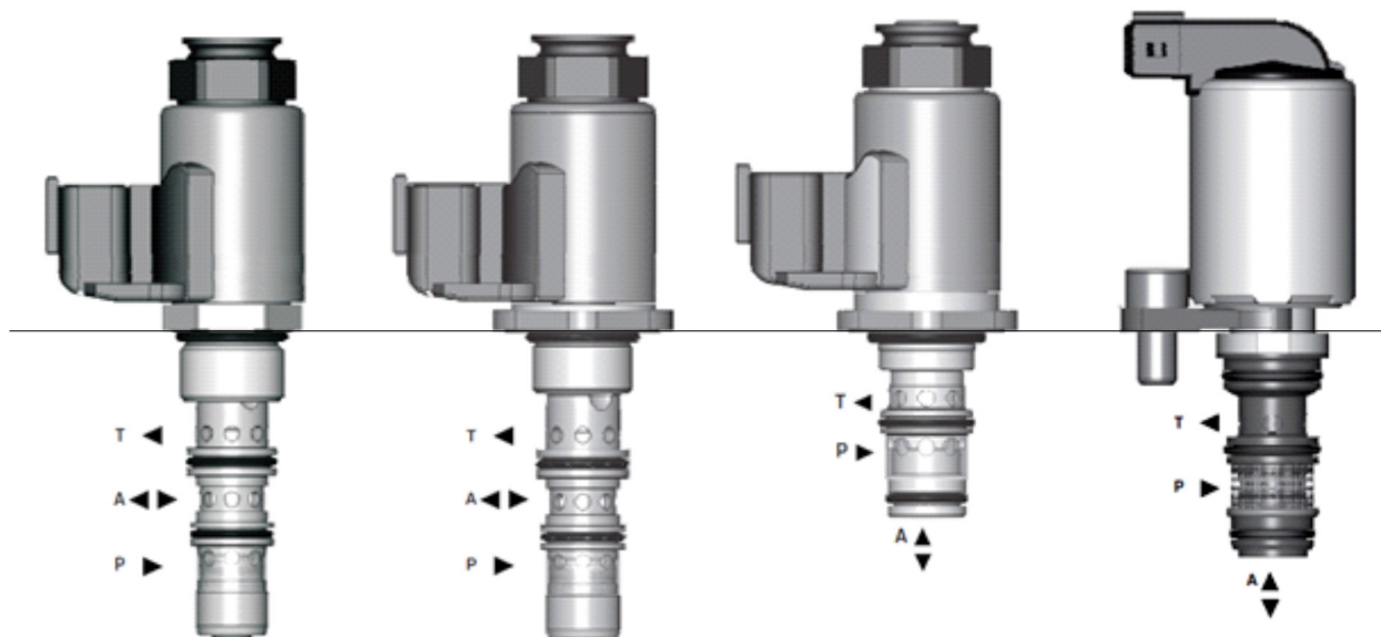
Vorgesteuertes Druckreduzier- und begrenzungsventil SP4P1-B4 mit 7/8-14 UNF Gewinde und Ventil PP4P1-Z3 als Einschubpatrone. Der Anschluss A verläuft in radialer Richtung.
