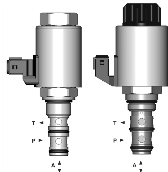
Die direktgesteuerten Druckreduzier- und begrenzventile PVRM1-063 and PVRM3-10 mit metrischem Gewinde.
