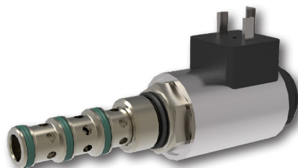
Eingebautes Wegeventil in Schieberausführung SD2E-B4/L - "Lightline"-Version
