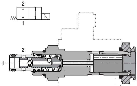
Eingebautes 2-Wege-Schieberwegeventil
