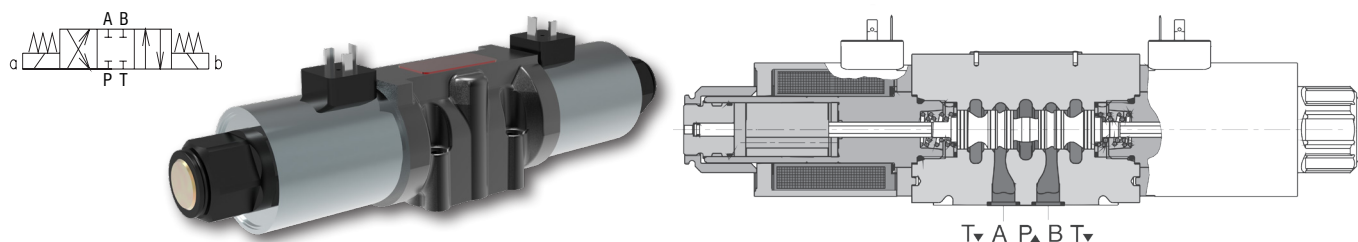
4-Wege-, 3-Positionenventil (4/3) mit zwei Stellmagneten
