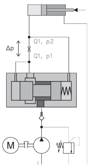
2-Wege Druckwaage compensator
