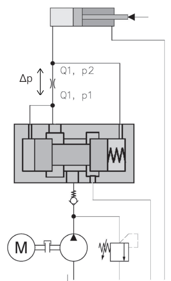
3-Wege Druckwaage
