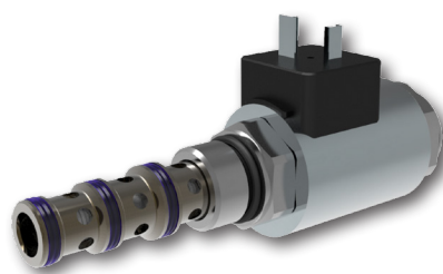
Eingebautes Wegeventil in Schieberausführung SD2E-B4
